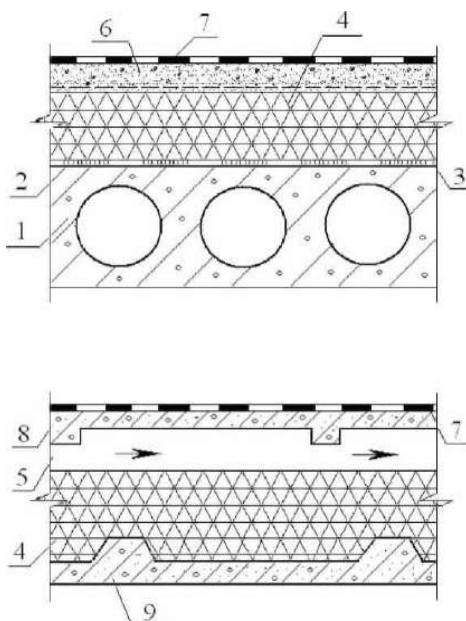
Рисунок 2 – Покрытия неветилируемых (а) и вентилируемых (б) бесчердачных крыш
