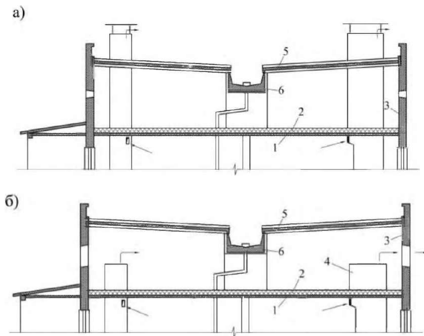
Рисунок 1 – Конструктивные схемы чердачных железобетонных крыш с безрулонной кровлей: а) с холодным чердаком; б) с открытым чердаком
