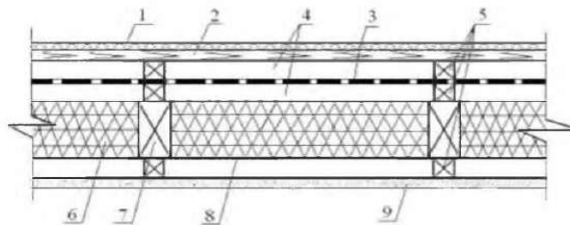
3-сүрөт – Бир (а) жана эки аба боштуктары бар жантайма чатырды (мансарда кабатынын үстүндө) куруу үчүн техникалык чечимдер.
