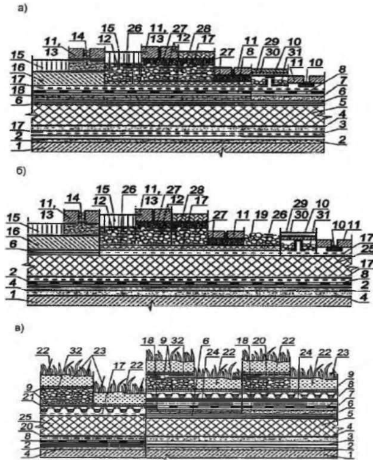
1б-сүрөт – Эксплуатацияланган, тескери жана жашылданган чатырлар үчүн конструктивдик чечимдер
