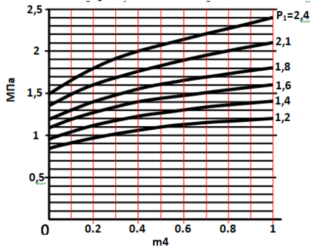
Рисунок Е.1 – График для определения давления в изотермическом резервуаре в конце выпуска расчетного количества двуокси углерода
