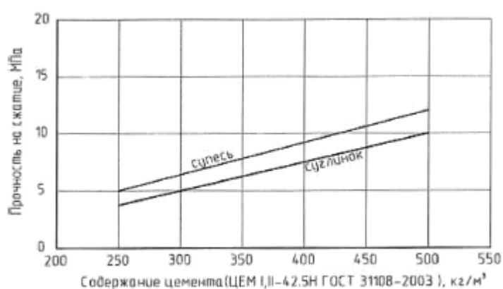
Рисунок Ф.3 – Зависимость прочности грунтоцемента от содержания цемента в 1 м 3 ГЦЭ
