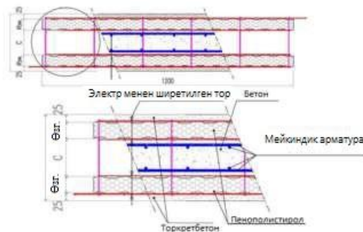
Г.2-сүрөт - Бекитилген электрширетилген болот торчолору менен эки пенополистриолдук такталардан турган кош панель
